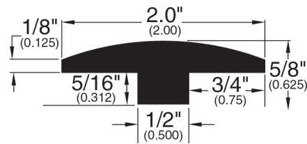
T-Mold (002)
